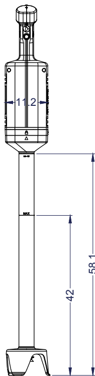
Vista Izquierda
