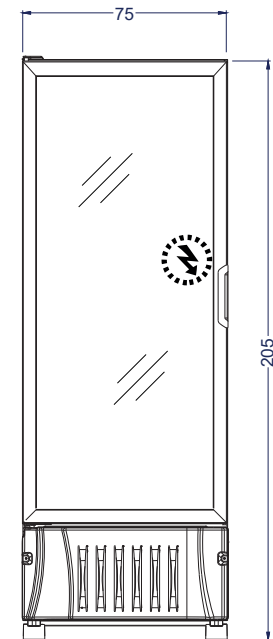
Vista Elevación
