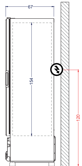
Vista Derecha
