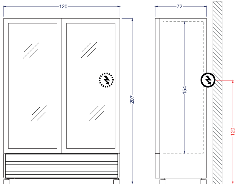
Vista Elevación
